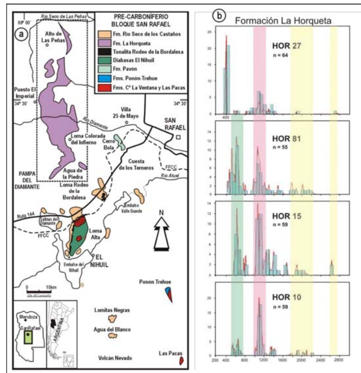
Figura 1: a) Representación esquemática de las unidades pre-Carboníferas del Bloque de San Rafael, Mendoza y ubicación de los afloramientos de la Fm. La Horqueta (modificado de González Díaz, 1981); b) Diagramas de frecuencias de edades U-Pb de circones detríticos y las diversas poblaciones reconocidas en cuatro muestras.
